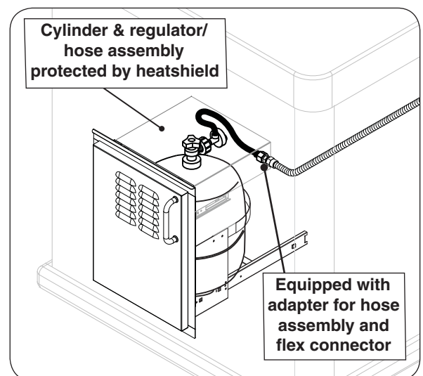
Fig. 11-3 Optional AOG door w/tank tray
